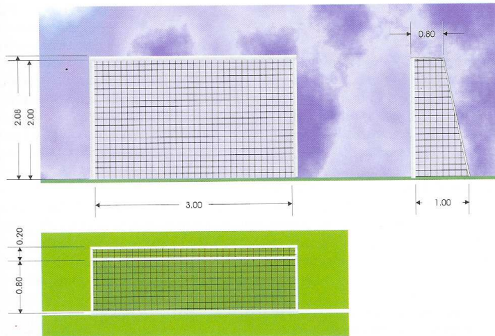
DIMENSIONI E PARTICOLARI DELLE PORTE DEL CALCIO A 5
