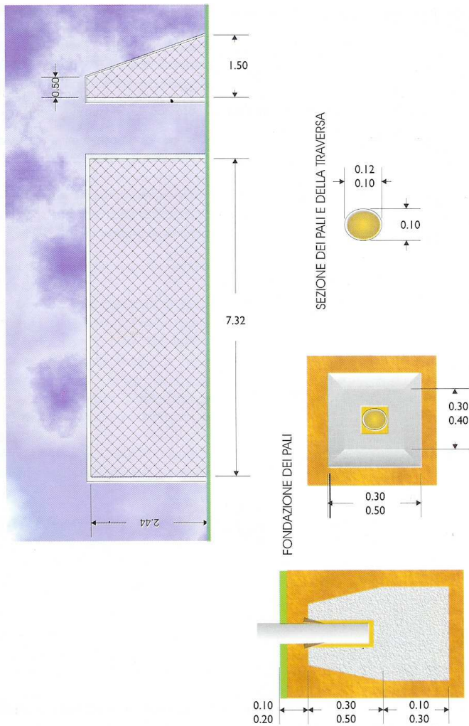
DIMENSIONI E PARTICOLARI DELLE PORTE
