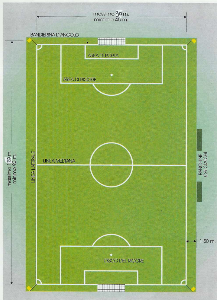
CAMPO DI CALCIO - DIMENSIONI GENERALI
